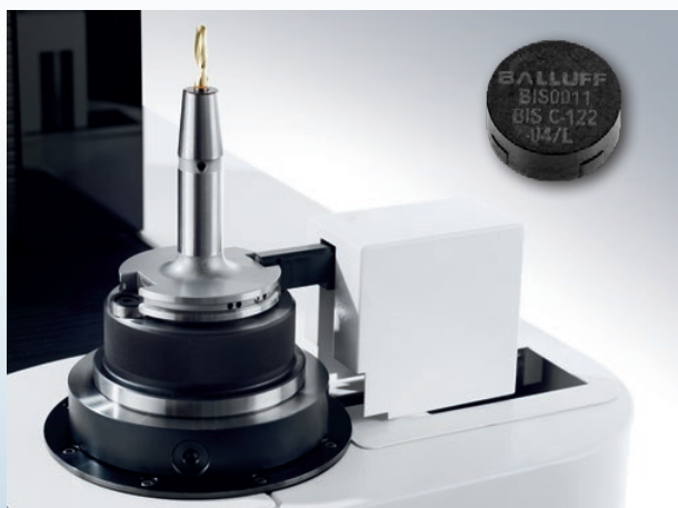
Nach dem Messen des Werkzeuges werden die Daten auf den Balluff Datenträger geschrieben/After measuring the tool, the data is transferred to the Balluff Chip
